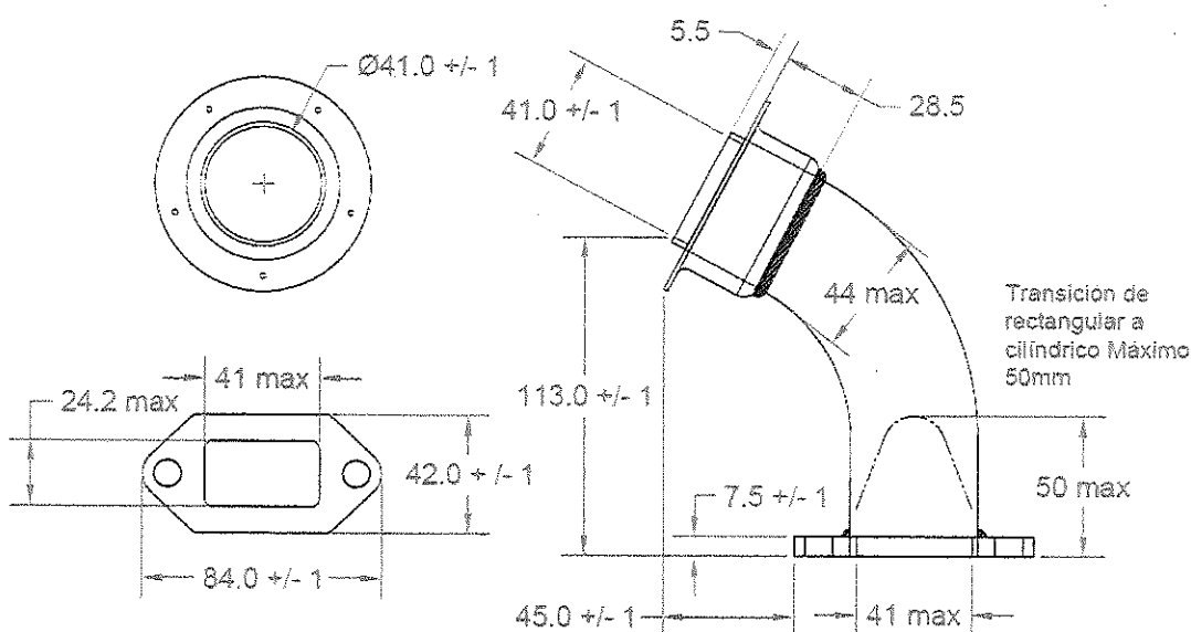
Figura 3-B cotas
