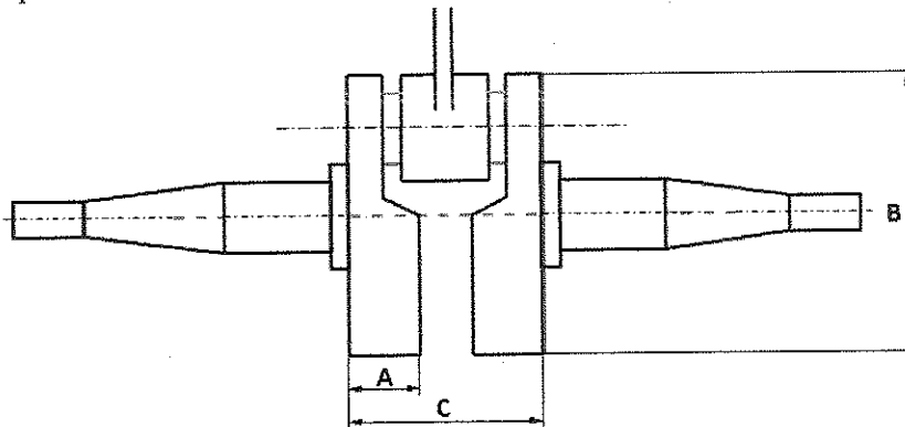
Figura 2 - Esquema de Cigüeñal
