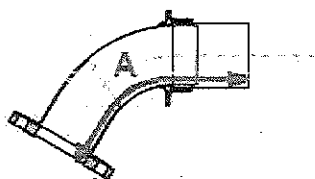
Figura 3 – Arco interior de coco de escape. 168mm \pm 2mm.
