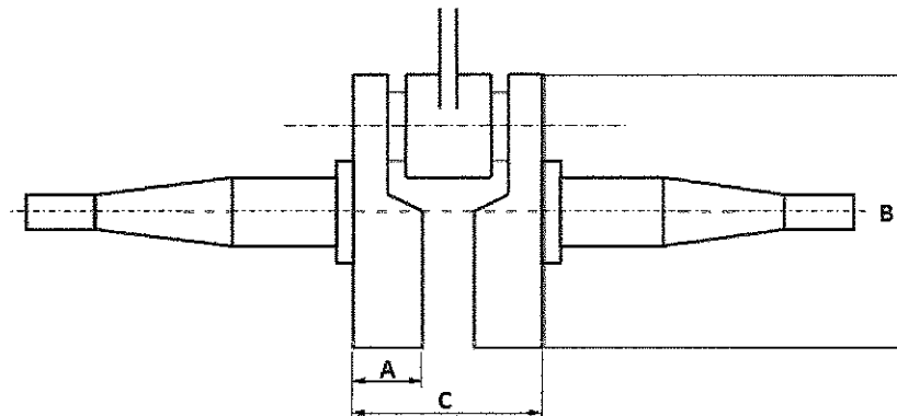
Figura 2 – Esquema y medidas del Cigüeñal
