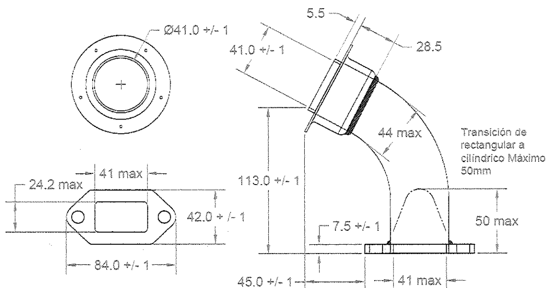
Figura 3-B cotas
