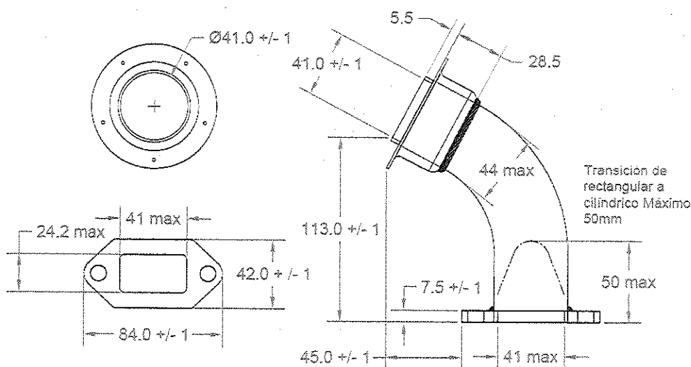
Figura 3-B cotas
