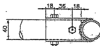
DIBUJO N° 253-34 Dimensiones en mm
